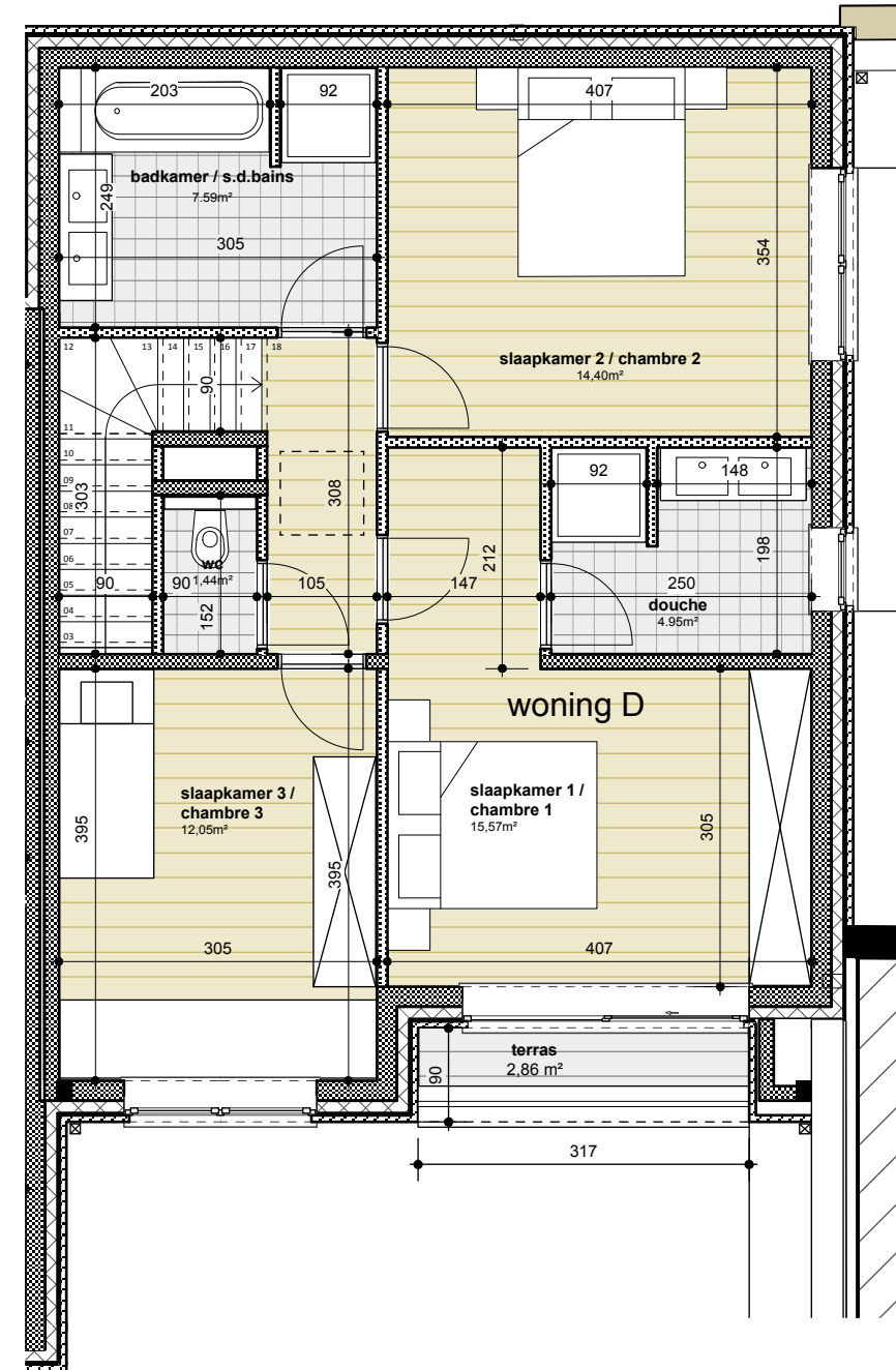
GRONDPLAN VERDIEPING
