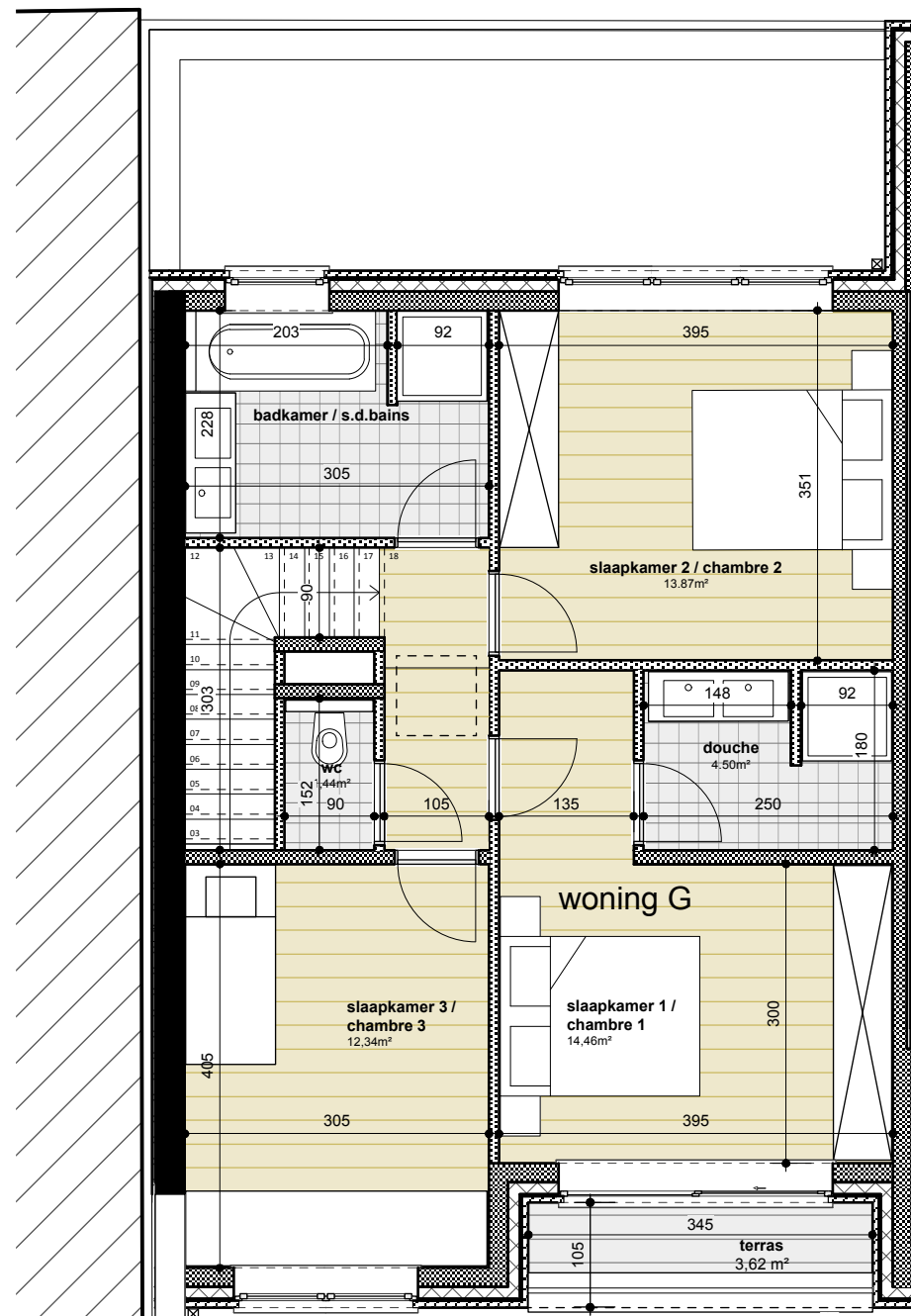
GRONDPLAN VERDIEPING
